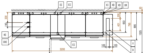
Boven aanzicht
