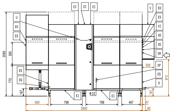
Zij aanzicht
